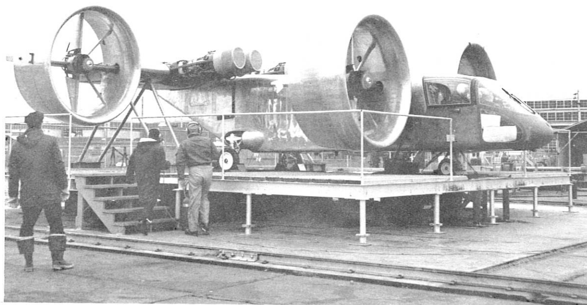
Tie-Down Test Stand
